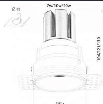
ГАБАРИТНАЯ СХЕМА
