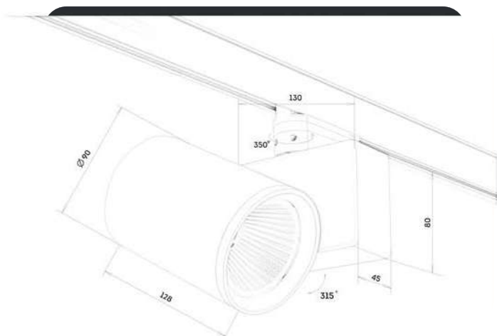
ГАБАРИТНАЯ СХЕМА
