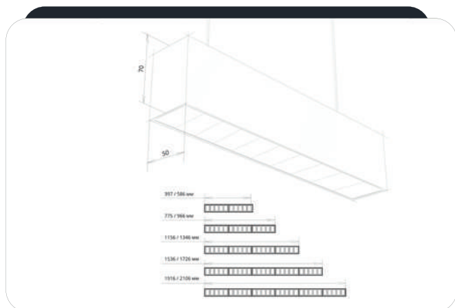
ГАБАРИТНАЯ СХЕМА
