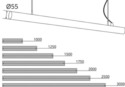
ГАБАРИТНАЯ СХЕМА
